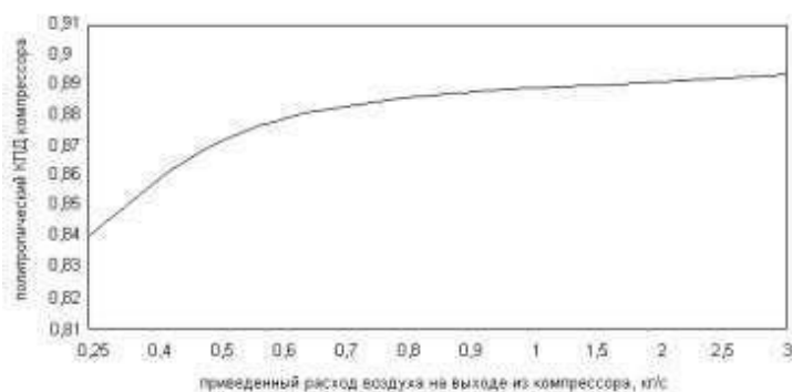
Рис.1. Зависимость политропического КПД осецентрибежного компрессора от приведенного расхода воздуха на выходе из двигателя
